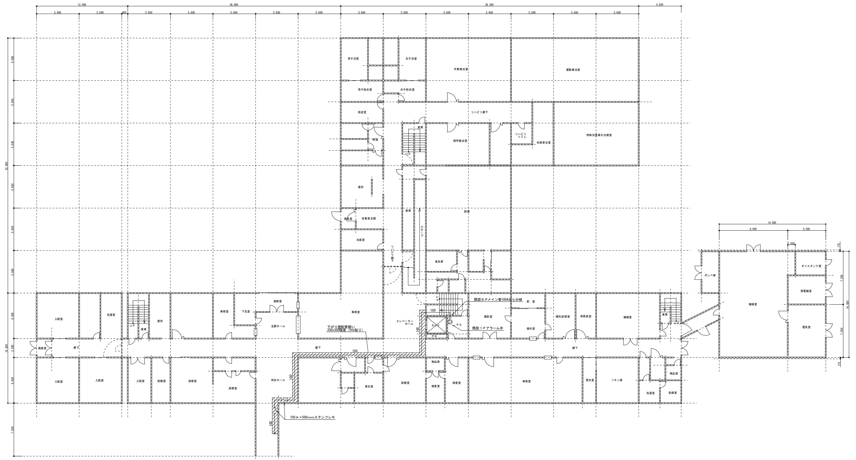
渡島リハビリテーションセンター1階平面図
